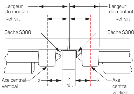
Figure 7 Paire de portes avec meneau
