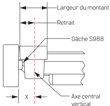
Figure 6 Porte simple et cadre en aluminium
