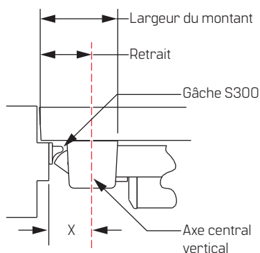
Figure 5 Porte métallique creuse simple
