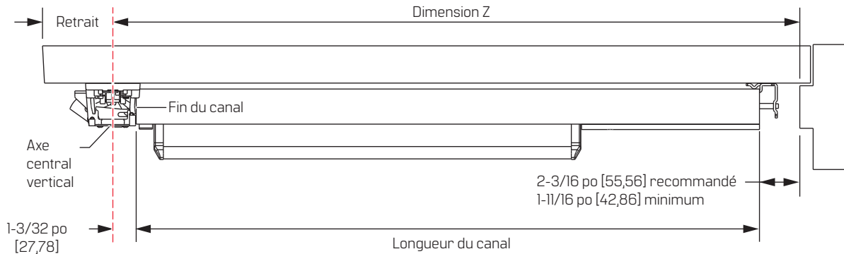
Figure 2 Schéma du dispositif
