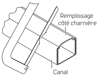
Figure 3 Coupe du dispositif
