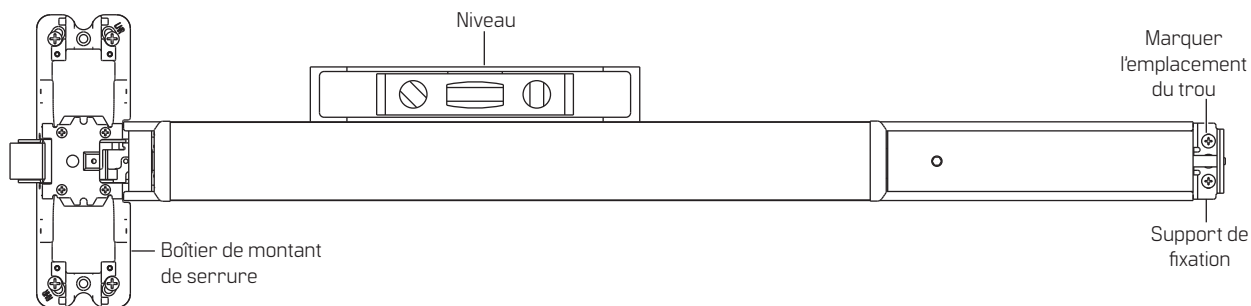
Figure 8 Dispositif de sortie en applique de la série 2 1 | FL 2 1 (ambidextre)
