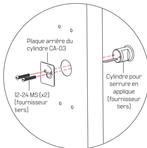
Figure 9 Installation du cylindre seul
