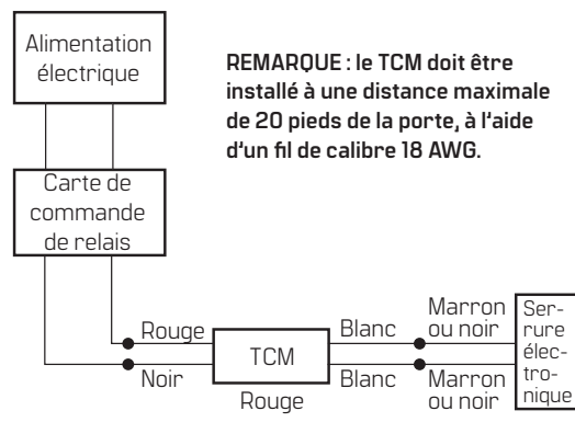
Figure 2 Schéma de câblage du TCM
