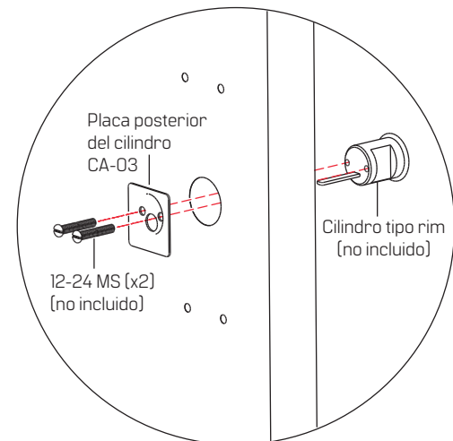
Figura 9 Instalación solo del cilindro
