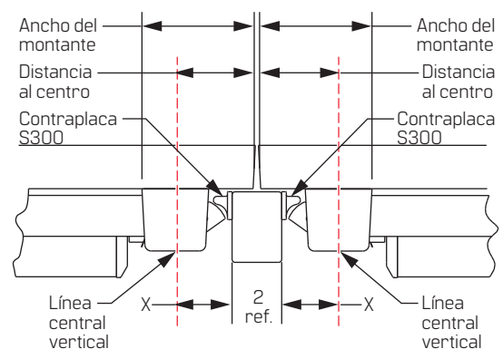
Figura 7 Puertas dobles con parteluz
