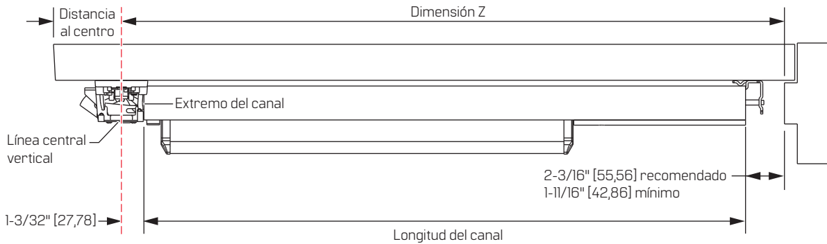
Figura 2 Esquema del dispositivo
