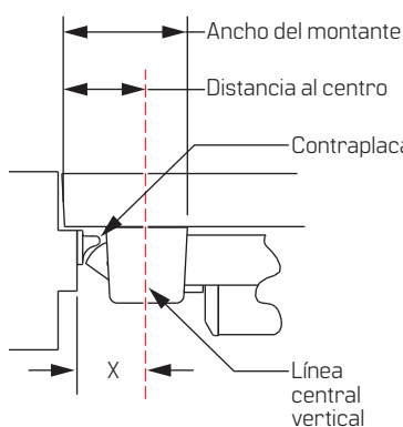
Figura 5 Puerta simple de metal hueco
