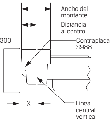
Figura 6 Puerta y marco simple de aluminio
