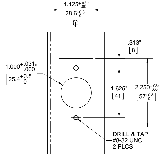
DOOR EDGE DETAIL
